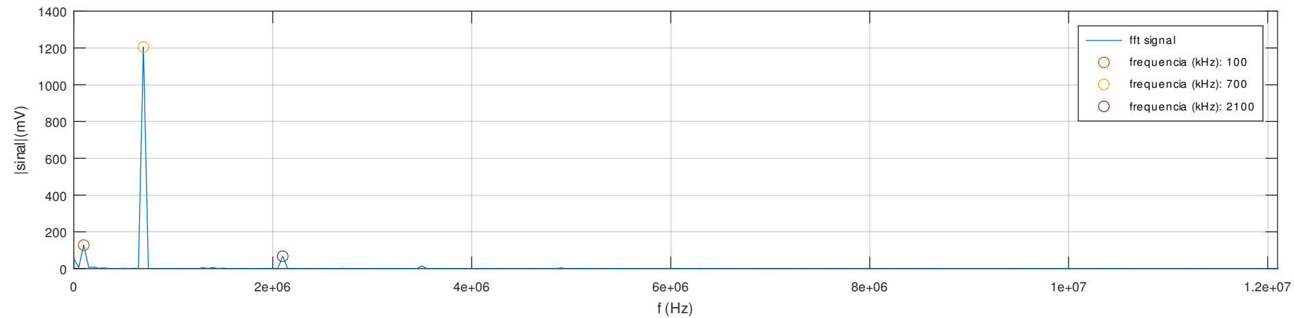
Espectro de amplitudes unilateral X(t) - Saída f=700\text{kHz} do gerador de sinais com ganho máximo
